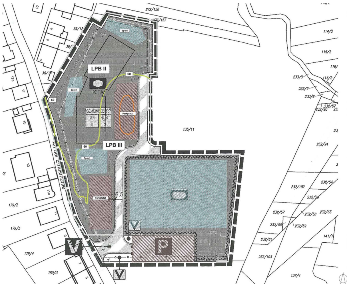
Lärmpegelbereiche nach DIN 4109 [2018], tags – Maßgeblicher Außenlärmpegel L_a in dB(A)
